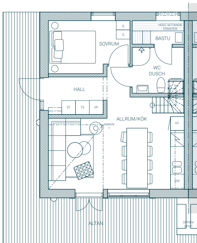
ENTRÉPLAN
