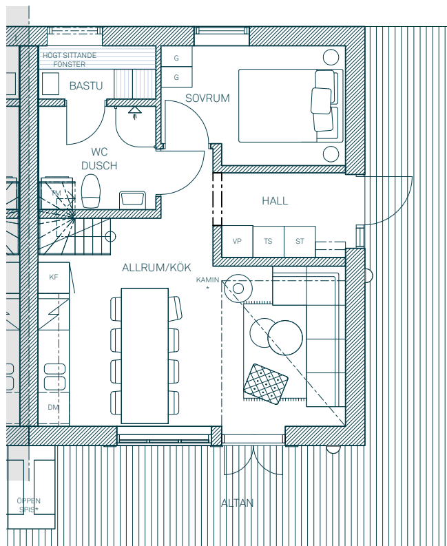
ENTRÉPLAN
