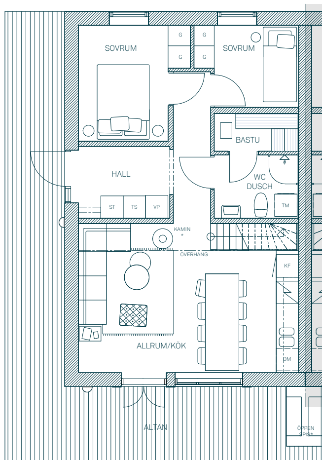
ENTRÉPLAN
