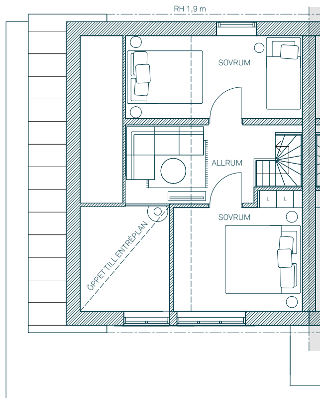
ÖVRE PLAN
